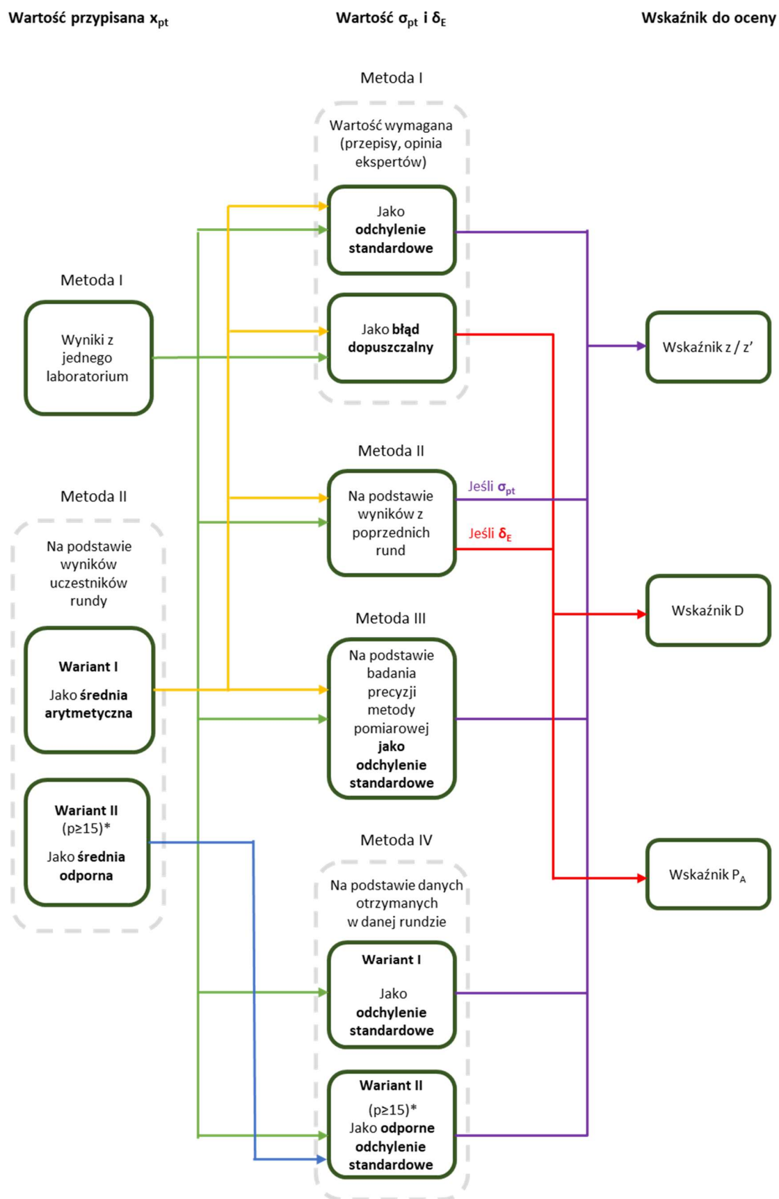
Rys. 2. Algorytm modelu statystycznego w badaniach biegłości
