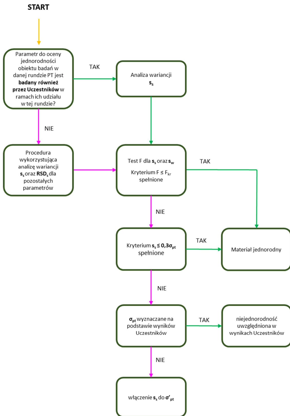
Rys. 1. Algorytm oceny jednorodności w badaniach biegłości
