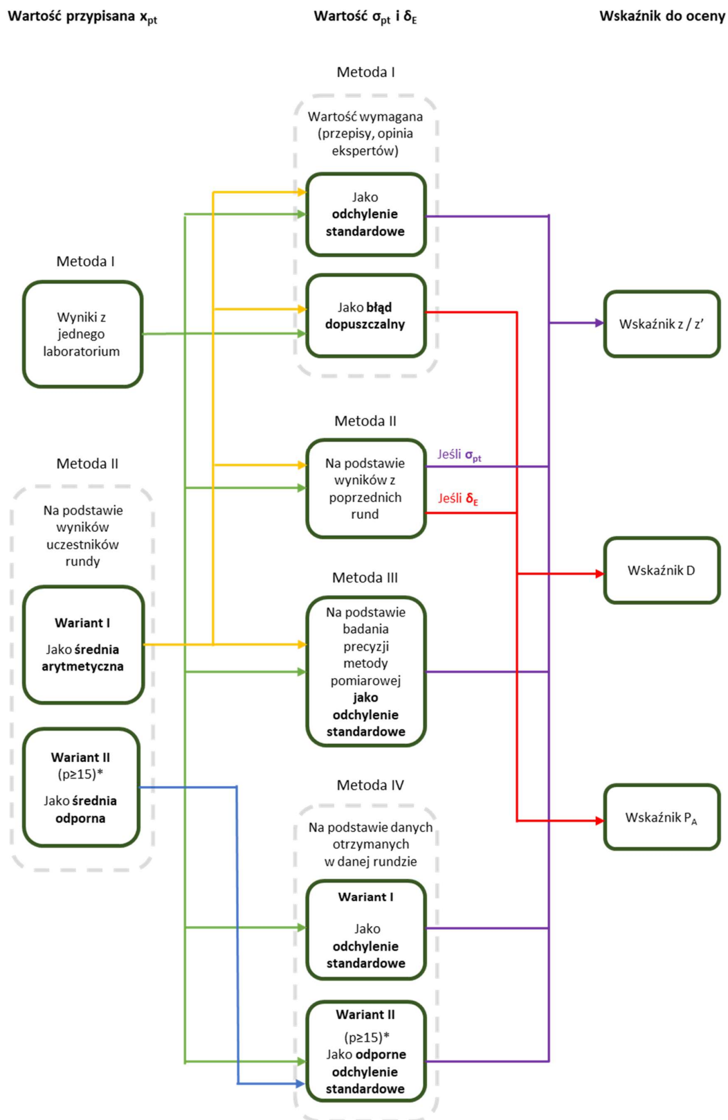
Rys. 3. Algorytm modelu statystycznego w badaniach biegłości
