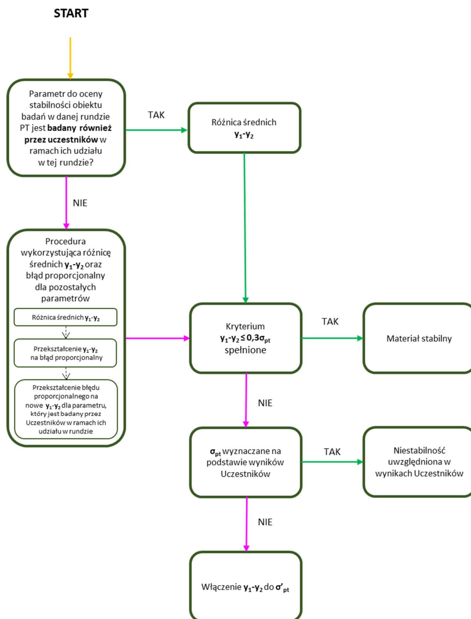
Rys. 2. Algorytm oceny stabilności w badaniu biegłości
